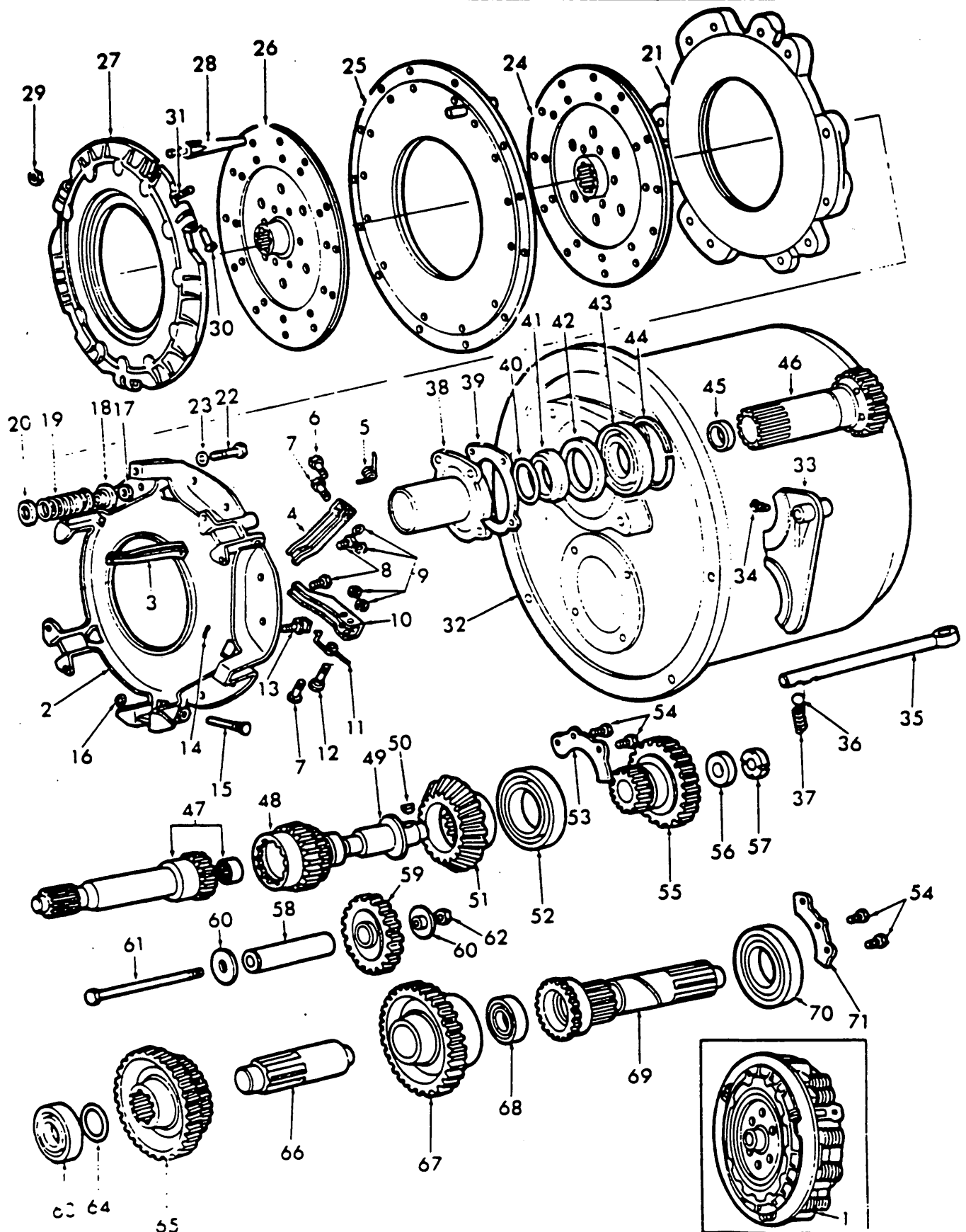
Fig. 53 - Clutch & Live PTO
