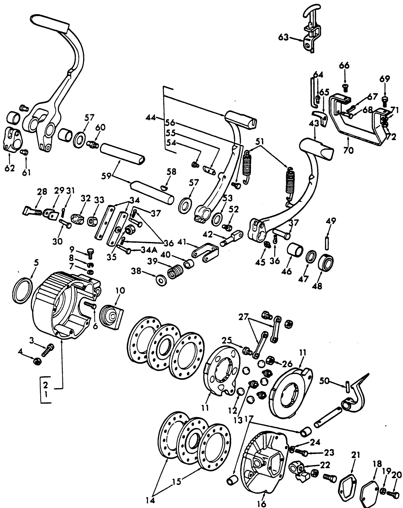
Fig. 7 - Steering Disc. Brakes 11-60/64
