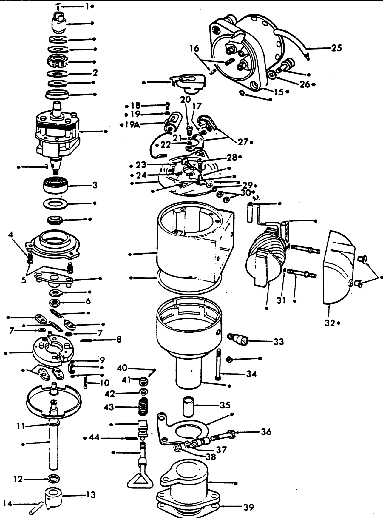
Fig. 82 - Magneto
