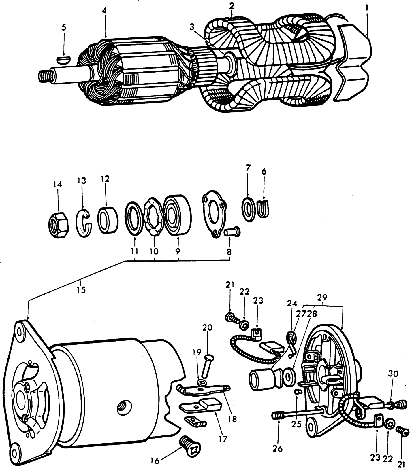
Fig. 85 - Generator
