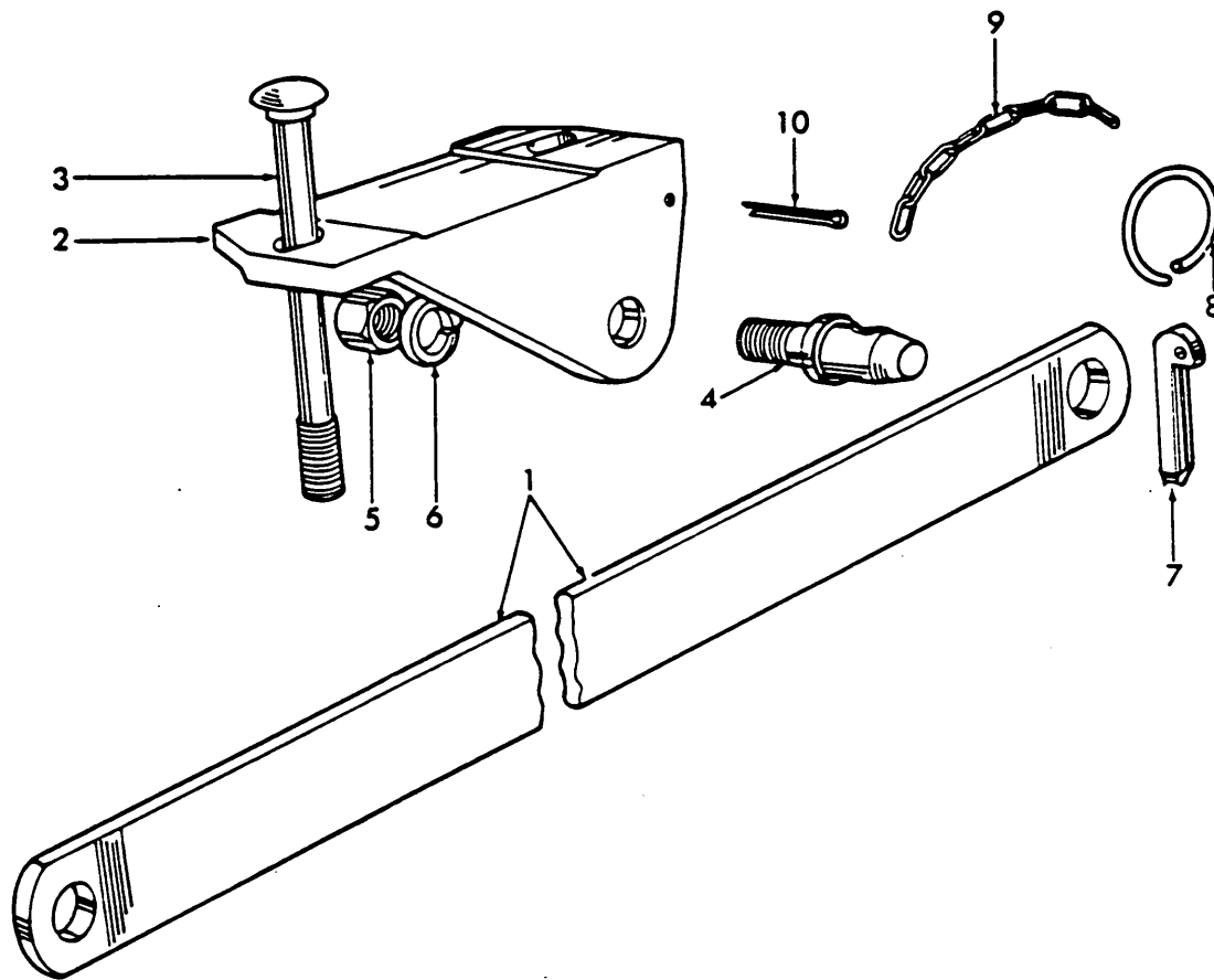
Fig. 15 H.P.L. Link Stabilizer
