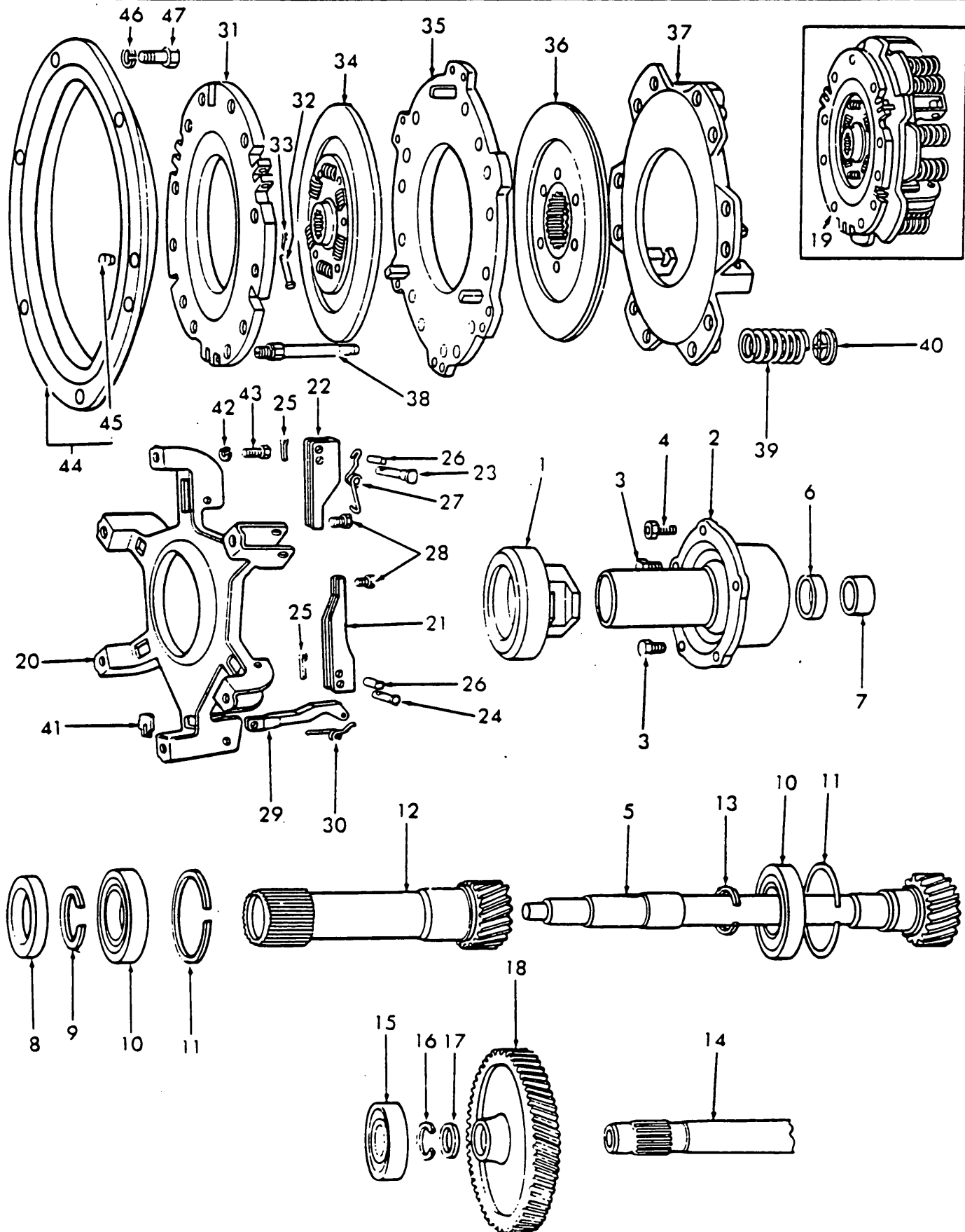
Fig. 50 Live P.T.O. & Clutch
