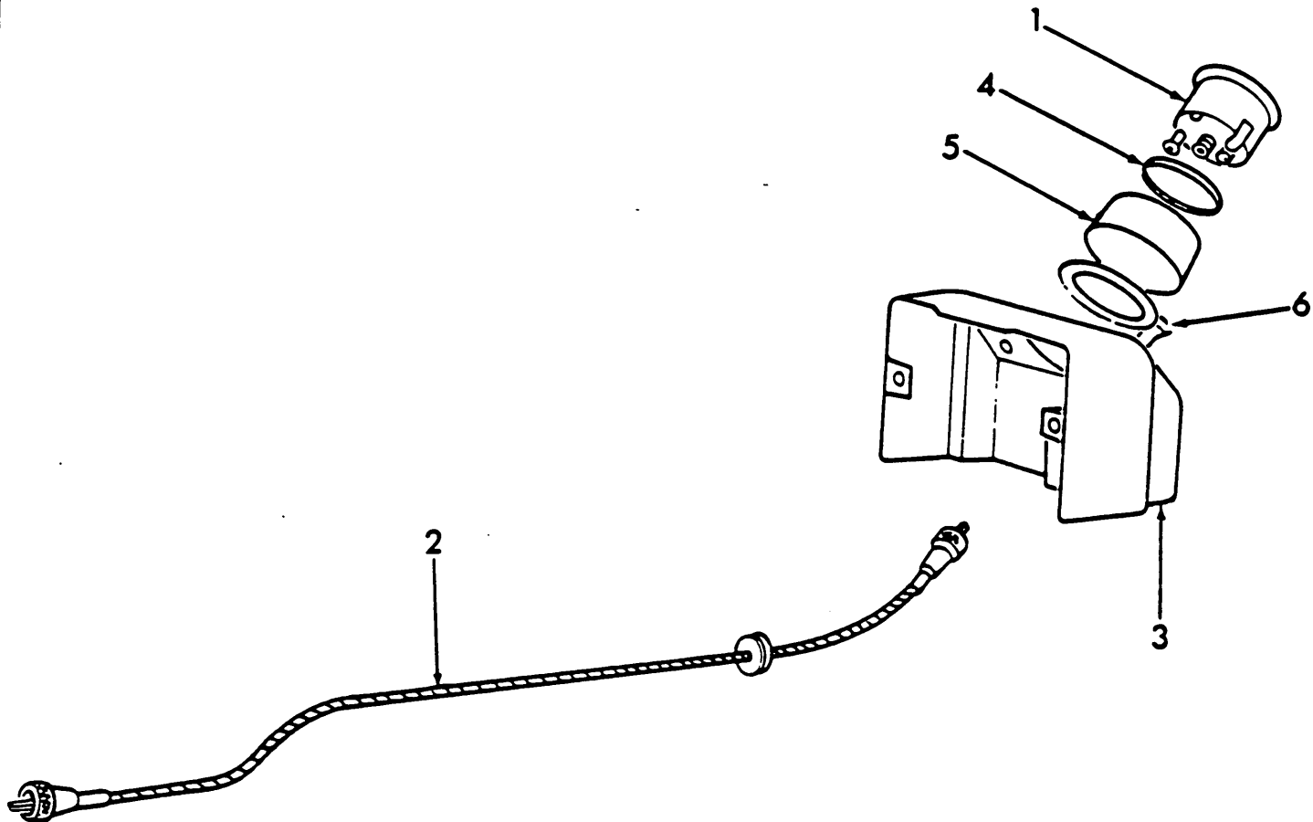
Fig. 53 Tachometer
