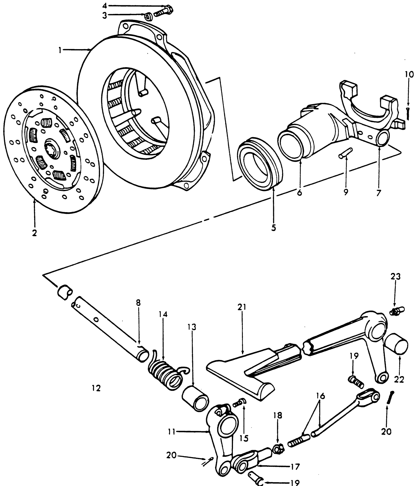
Fig. 31 Clutch & Linkage
