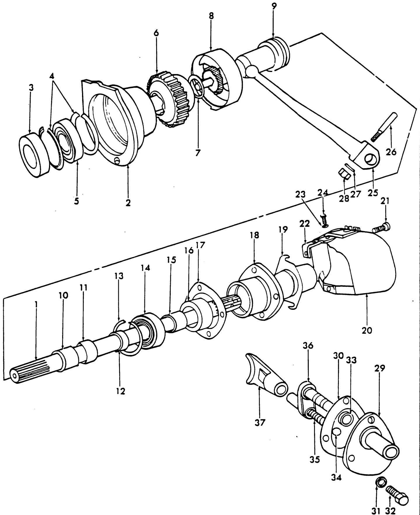
Fig. 29 Standard P.T.O.
